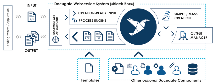
Abbildung 1: Auszug aus dem Docugate Applikationsschema für "Docugate Webservice System"
